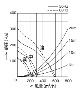
静圧－風量 曲線
