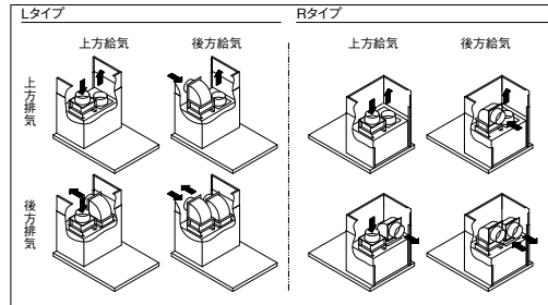
排気パターン
