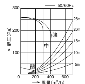
静圧－風量 曲線
