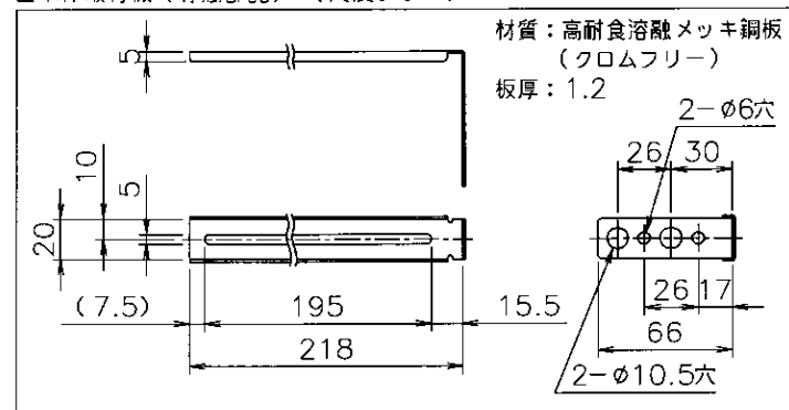
■本体取付板（付属部品）（尺度フリー）
