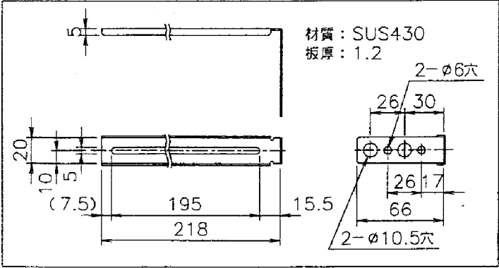
■本体取付板（付属品）（尺度：フリー）
