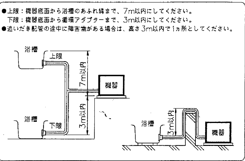
■追いただき配管工事＜最大延長は、片道15m10曲がり（φ12.7銅管の場合）です。
