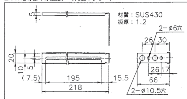
■本体取付板（付属品）（尺度：フリー）
