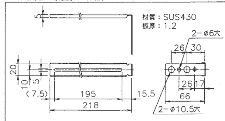
■本体取付板（付属品）（尺度：フリー）
